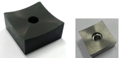
Faca para Trituradores Mono Eixo Incluindo Retífica e Tempera
